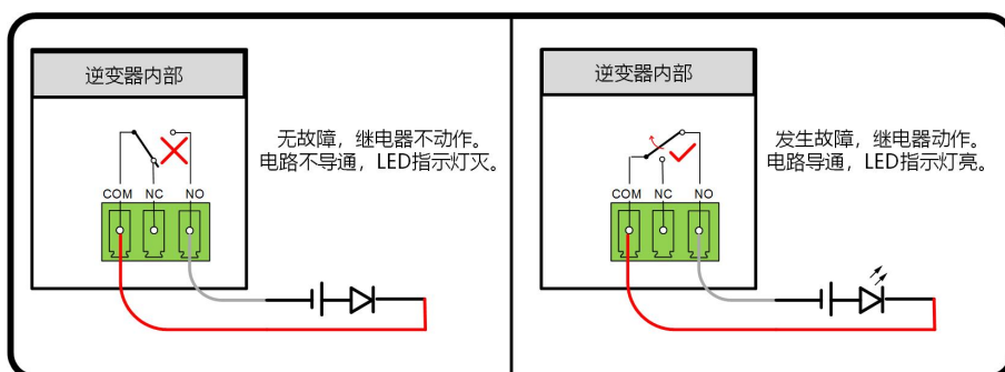
图 5-6 设置为常开触点
