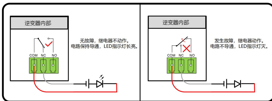
图 5-7 设置为常闭触点
