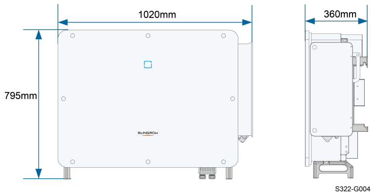
图 2-3 产品尺寸（单位：mm）
