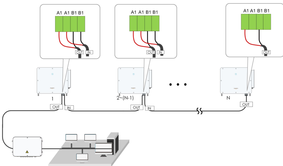
图 5-5 多台逆变器通讯系统
