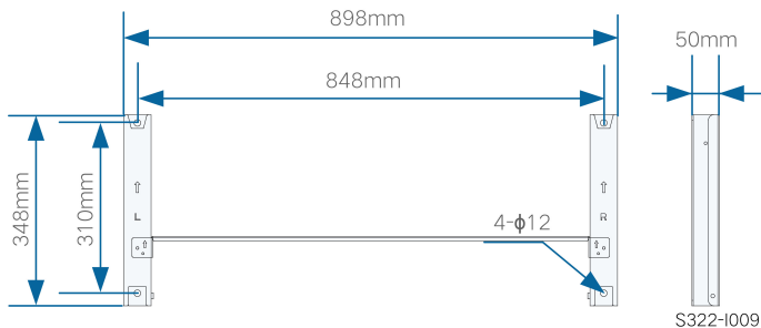
图 4-1 挂板尺寸
