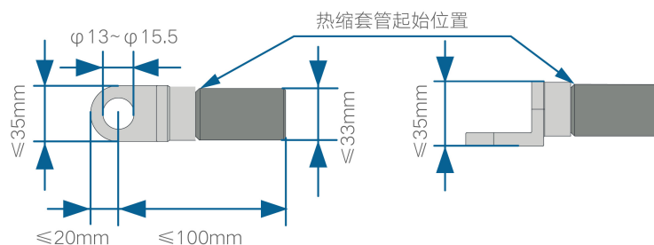
图 5-3 端子压接后尺寸
