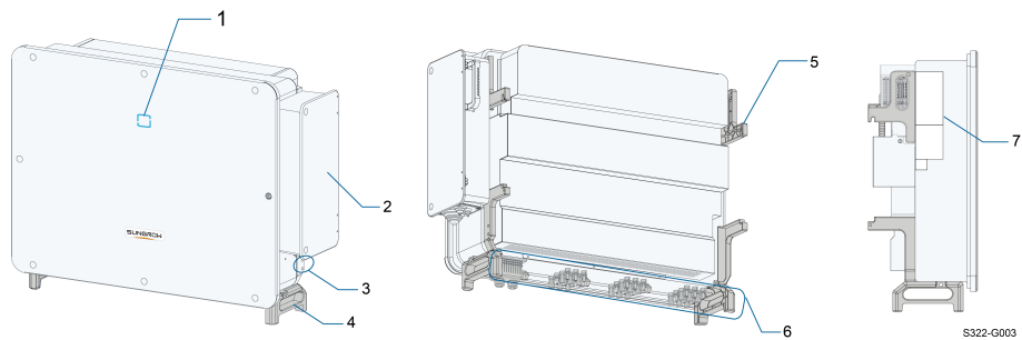
图 2-2 产品外观
