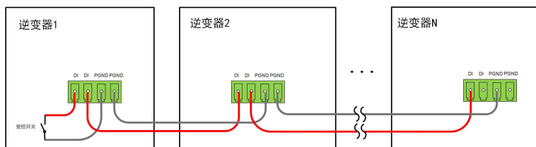
图 5-9 多台逆变器连接成菊花链式拓扑
