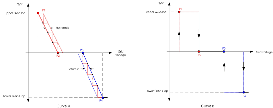
图 7-16 Q(U) 曲线
