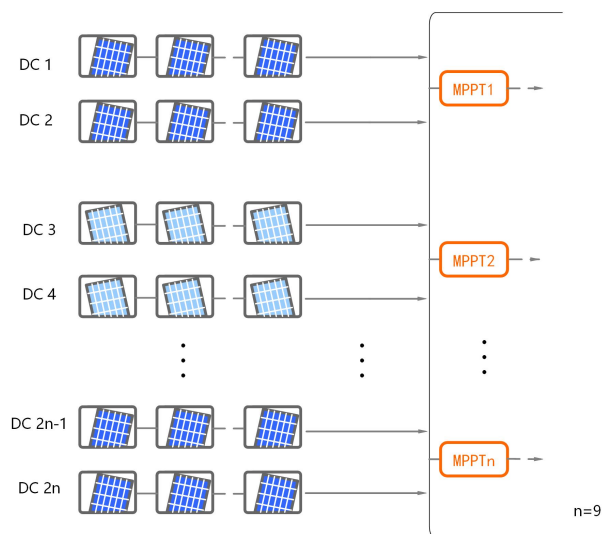
图 5-4 光伏输入配置
