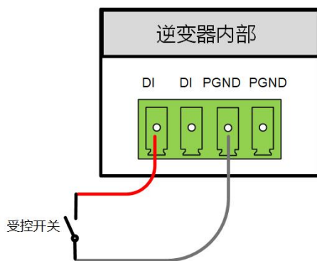
图 5-8 本地停止干接点典型应用
